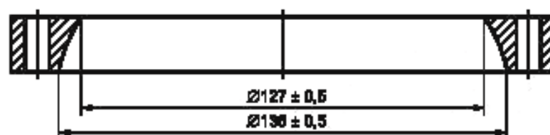
Рисунок 2 — Прижимное кольцо
