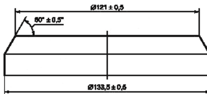
Рисунок 1 — Столик для истирания
