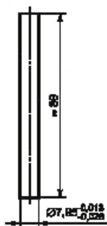
Рисунок 3 — Ось держателя пробы
