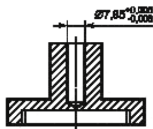
Рисунок 4 — Основание держателя пробы
