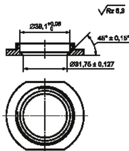
Рисунок 6 — Гайка держателя пробы
