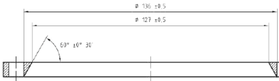
Рисунок 2 – Прижимное кольцо
