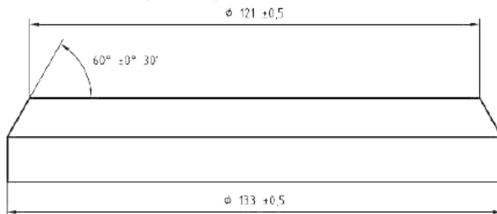
Рисунок 1 – Столик для истирания
