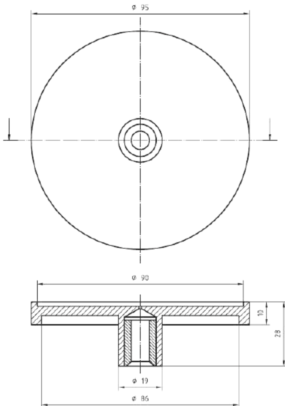
Рисунок 3 – Основание держателя пробы
