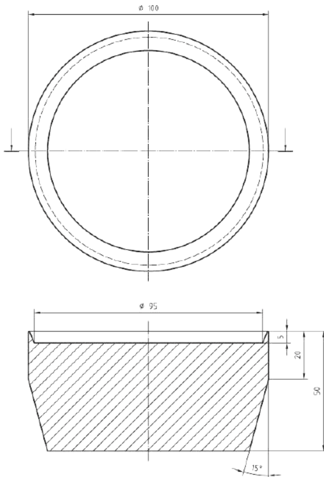
Рисунок 5 – Дополнительное устройство для установки проб
