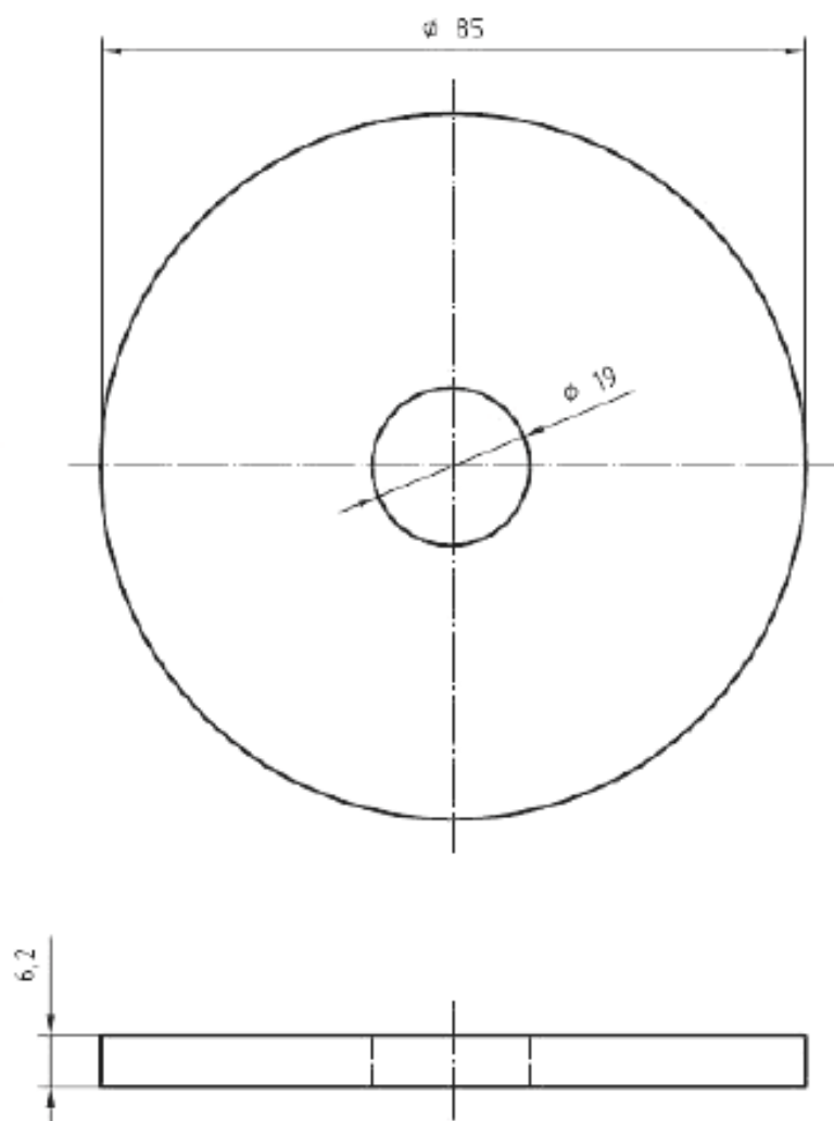
Рисунок 4 – Дополнительный груз
