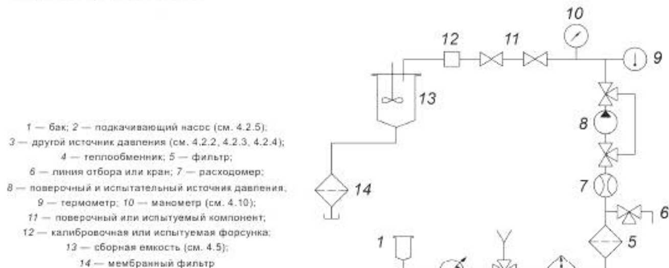
Рисунок А.1 — Принципиальная схема испытательной установки
