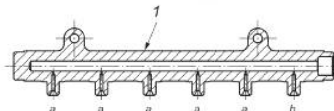
Рисунок В.1 — Аккумулятор перед испытанием
