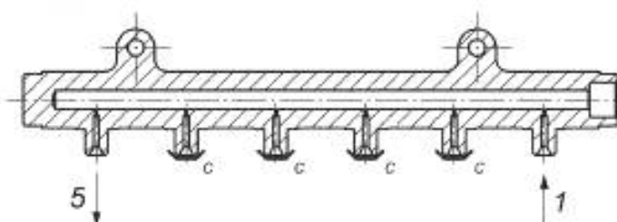
Рисунок В.1 — Аккумулятор перед испытанием
