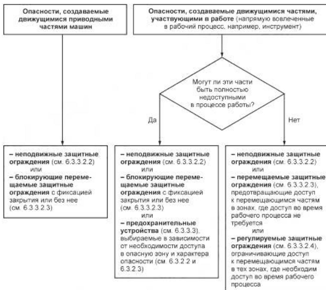
Рисунок 4 — Рекомендации по выбору защитных ограждений и предохранительных устройств, защищающих от опасностей, создаваемых движущимися частями машин
