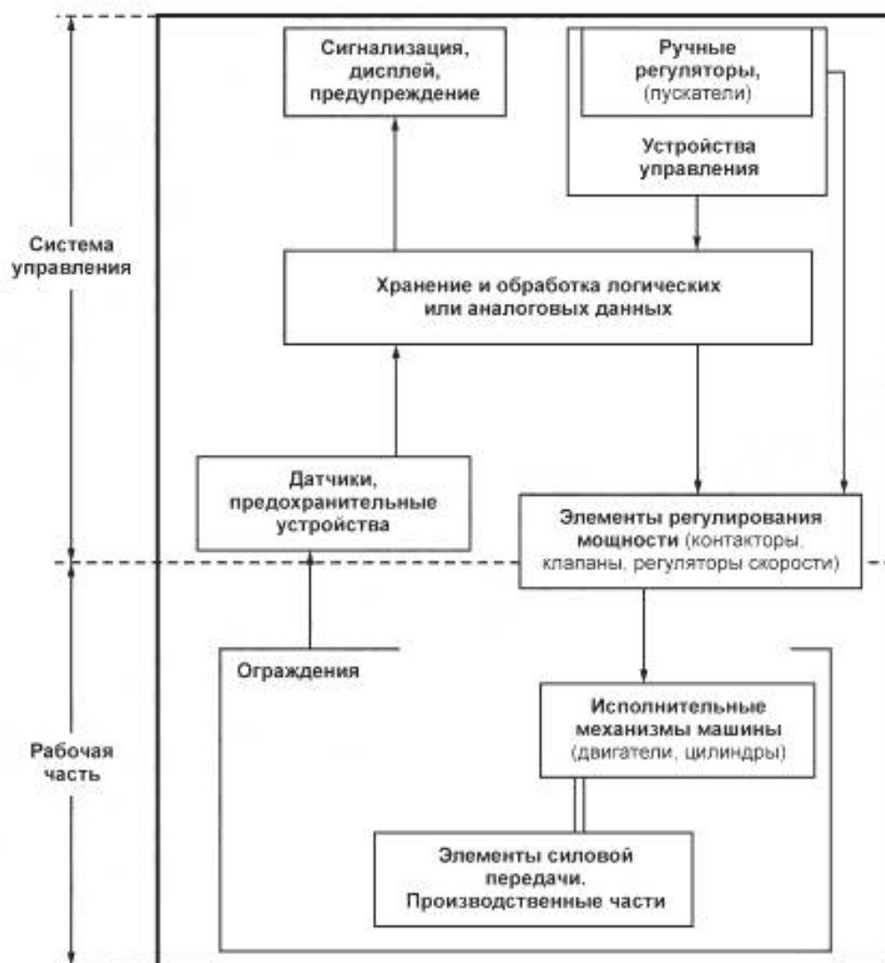
Рисунок А.1 — Общее схематическое изображение машины
