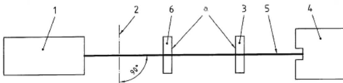
1 – лазер; 2 – опорная (референтная) ось; 3 – поляризатор; 4 – приемник излучения; 5 – лазерный пучок; 6 – четвертьволновая пластина; а – вращение в пределах 180^\circ
