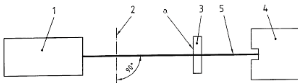
1 – лазер; 2 – опорная (референтная) ось; 3 – поляризатор; 4 – приемник излучения; 5 – лазерный пучок; а – вращение в пределах 180^\circ
