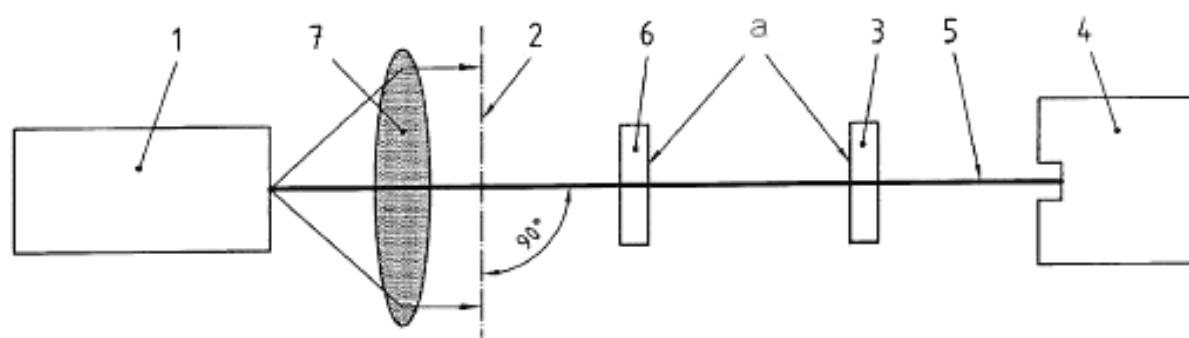
1 – лазер; 2 – опорная (референтная) ось; 3 – поляризатор; 4 – приемник излучения; 5 – лазерный пучок; 6 – четвертьволновая пластина; 7 – коллиматор; a – вращение в пределах 180^\circ
