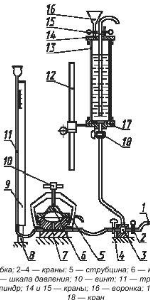
Рисунок 3 — Прибор типа Шоппера для оценки водопроницаемости
