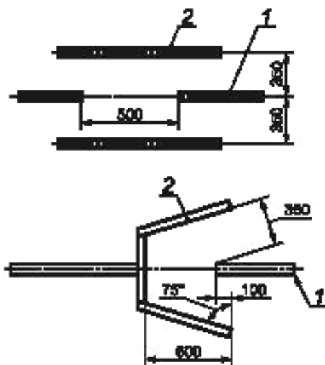
Рисунок Б.2 — Проход в ограждении
