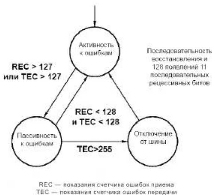
Рисунок 16 — Схема смены состояния узла
