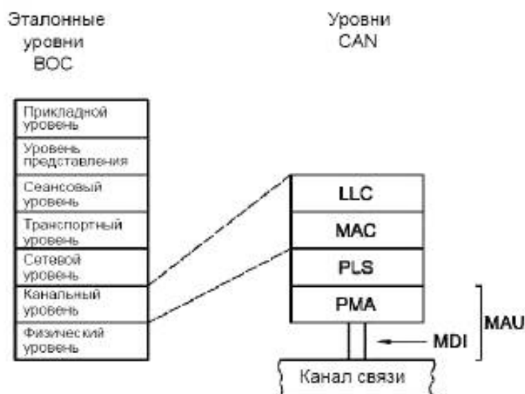
Рисунок 12 — Модель архитектуры физического уровня
