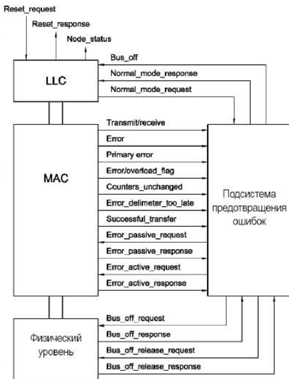
Рисунок 15 — Интерфейс предотвращения ошибок
