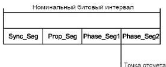
Рисунок 13 — Разделение битового интервала
