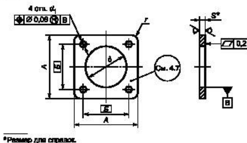
Рисунок 2 — Держатель ДП
