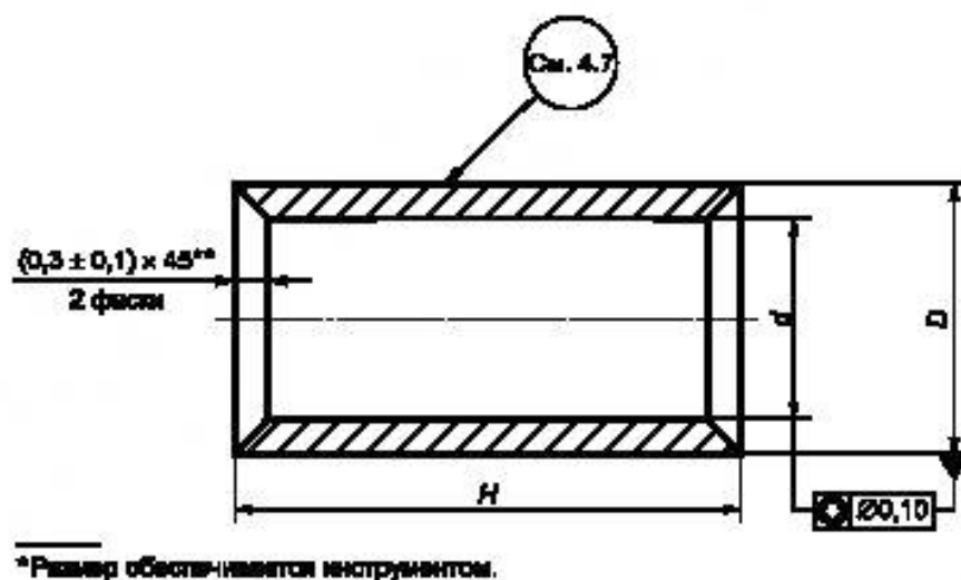
Рисунок 1 — Конструкция втулок
