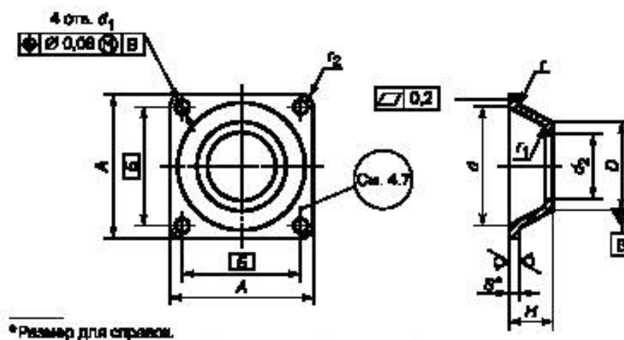
Рисунок 3 — Держатель ДЧ
