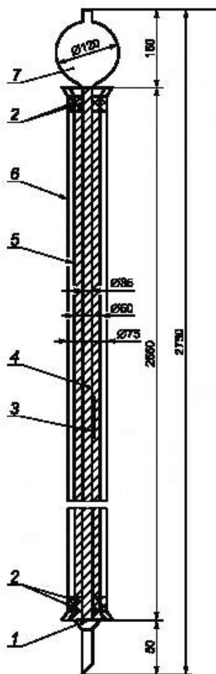
1 — стеклянная вата; 2 — асбестовый уплотнитель; 3 — термометр; 4 — адсорбционная колонка; 5 — внутренняя трубка муфты со спиралью из никромовой проволоки; 6 — внешняя трубка муфты; 7 — резервуар для налива испытуемого продукта
