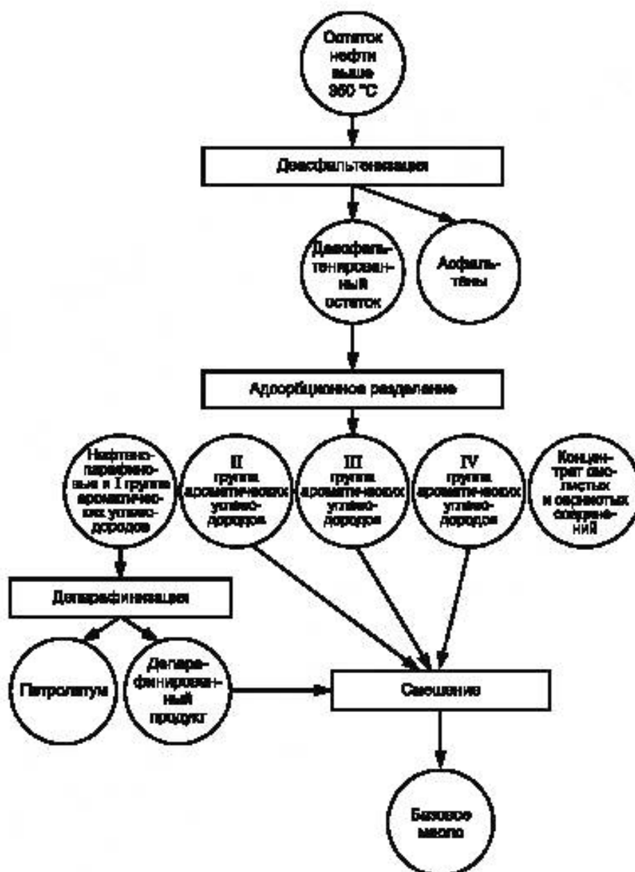
Рисунок 5 — Схема испытаний остатка нефти при температуре от 350 °C до 480 °C
