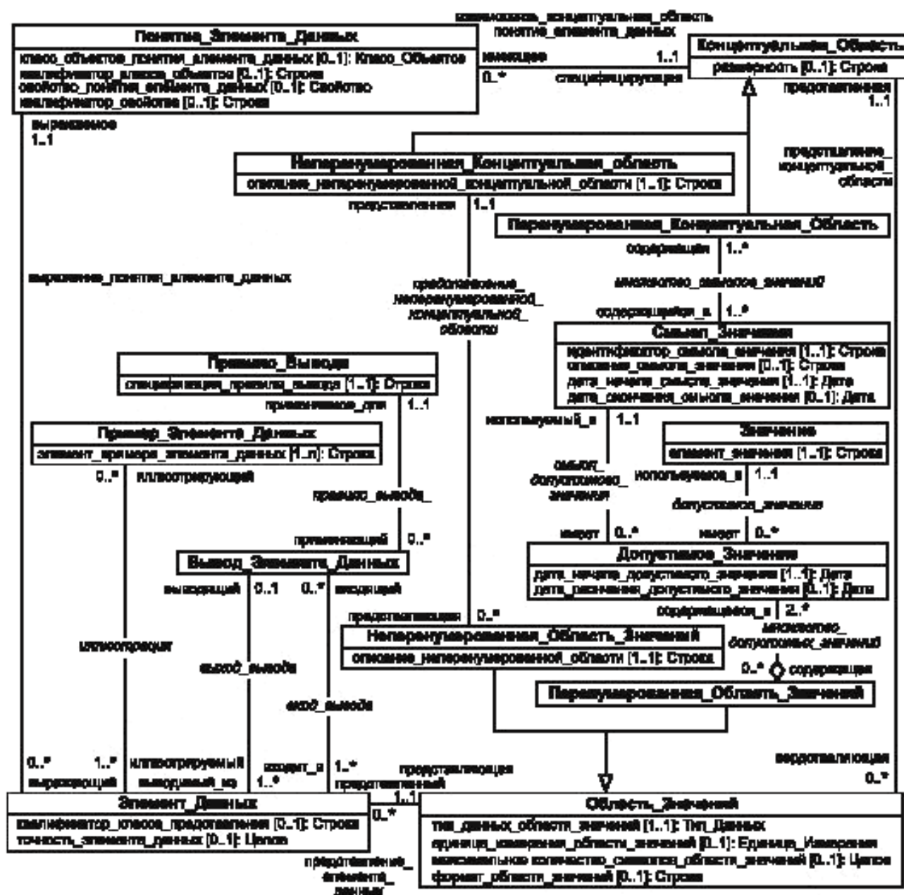
Рисунок 11 — Консолидированная метамодель
