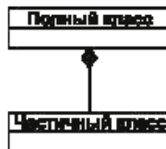
Рисунок В.9 — Нотация для составной агрегации
