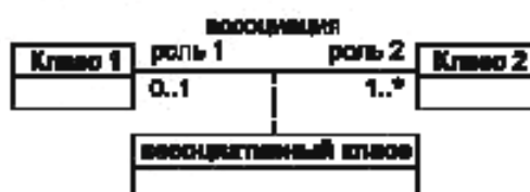
Рисунок В.6 — Нотация для ассоциативного класса
