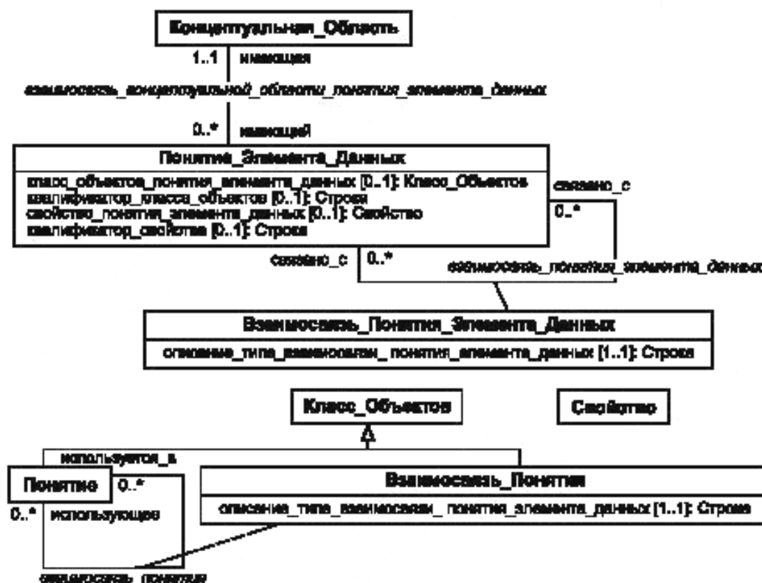
Рисунок 8 — Область Понятий Элементов данных метамодели (Cor.1:2004)
