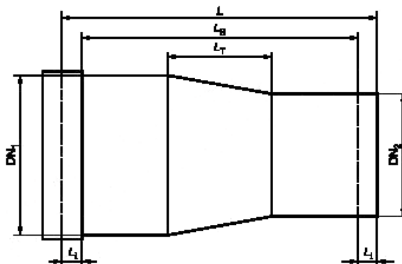
а — Переходник с концентричным расположением концевых отверстий
