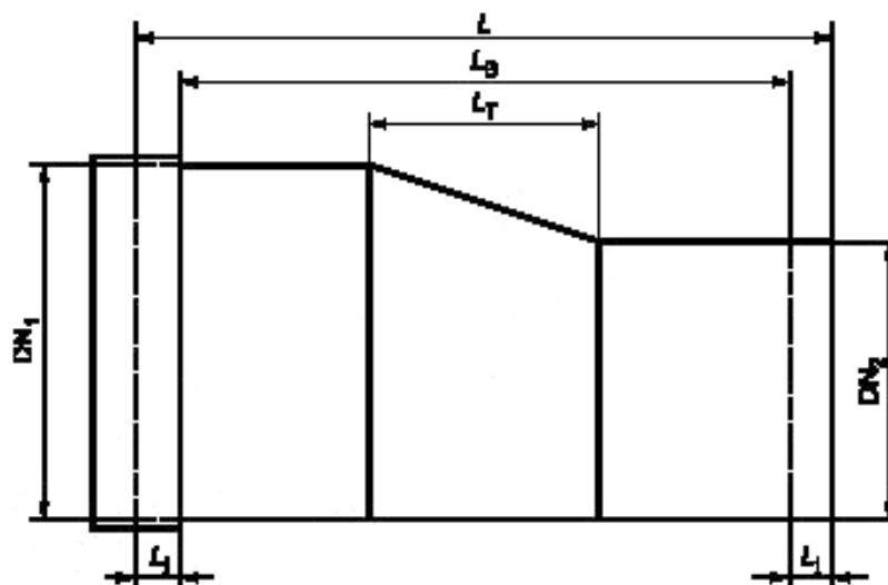
б — Переходник с эксцентричным расположением концевых отверстий
