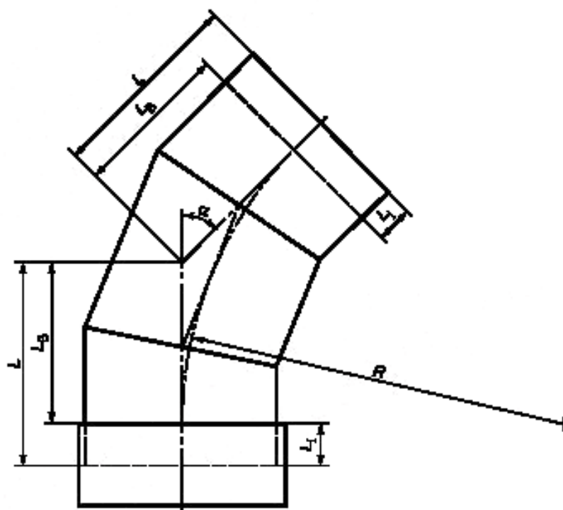
Рисунок 2 — Пример литого отвода
