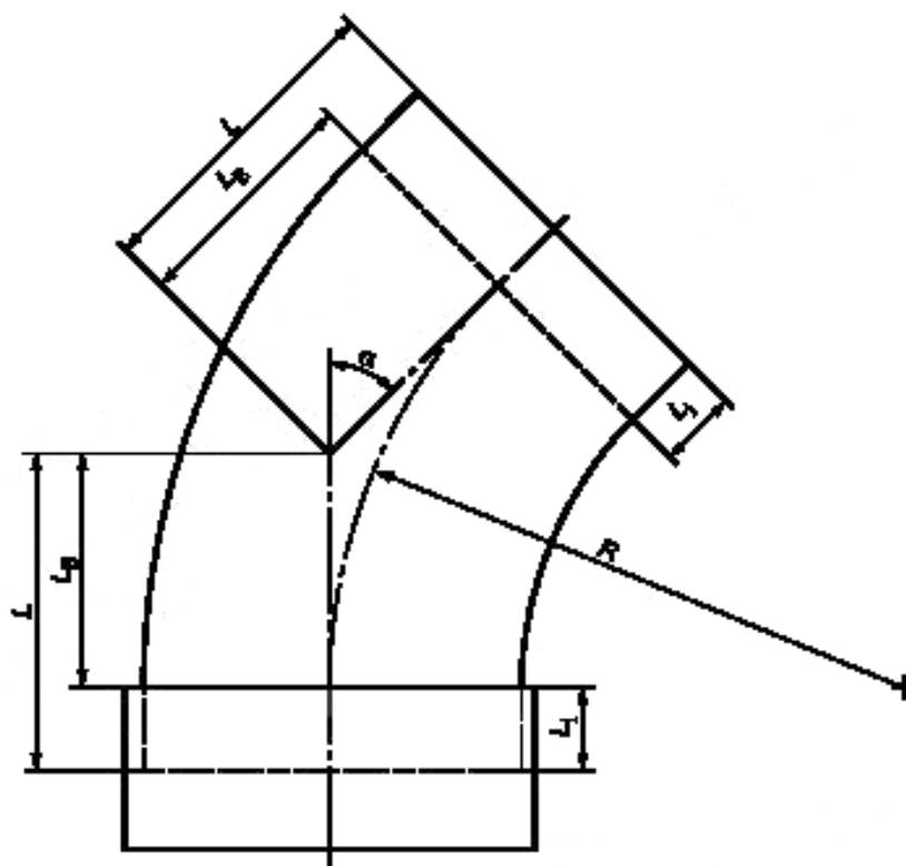
Рисунок 2 — Пример литого отвода
