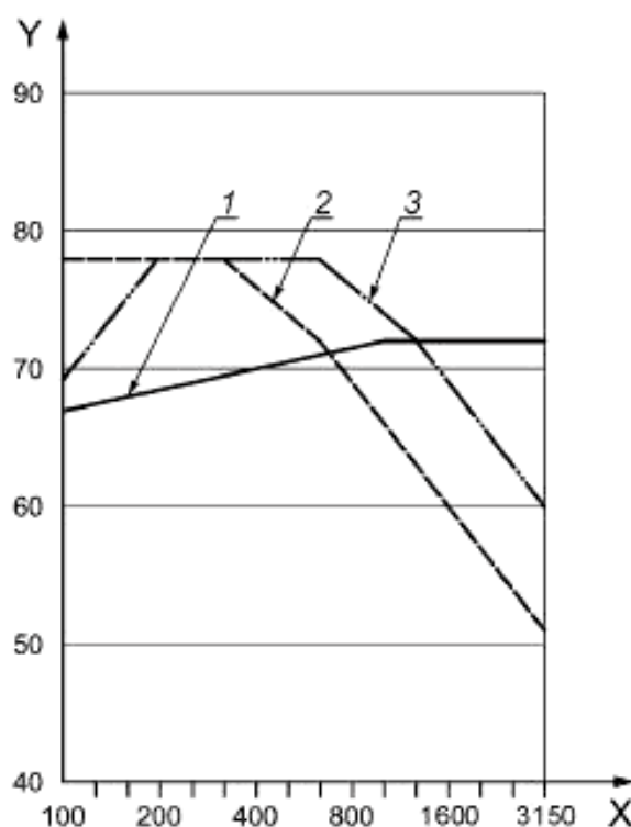
Рисунок С.5 — Частотные характеристики приведенного уровня звукового давления ударного шума L_p стандартных полов
