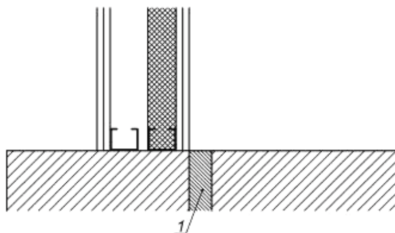
1 — обрамление испытательного проема
