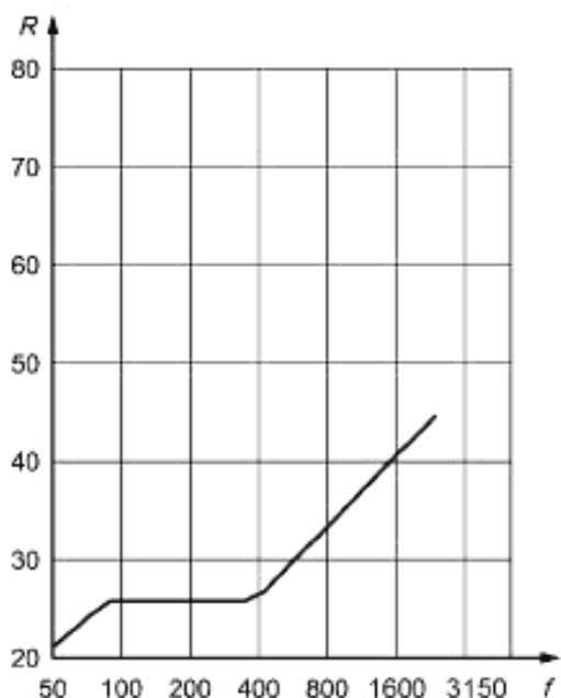
Рисунок В.3 — Частотная характеристика звукоизоляции стандартной стены со средней критической частотой
