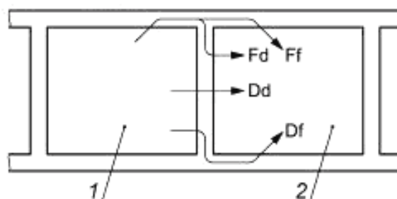
1 — помещение источника; 2 — приемное помещение
