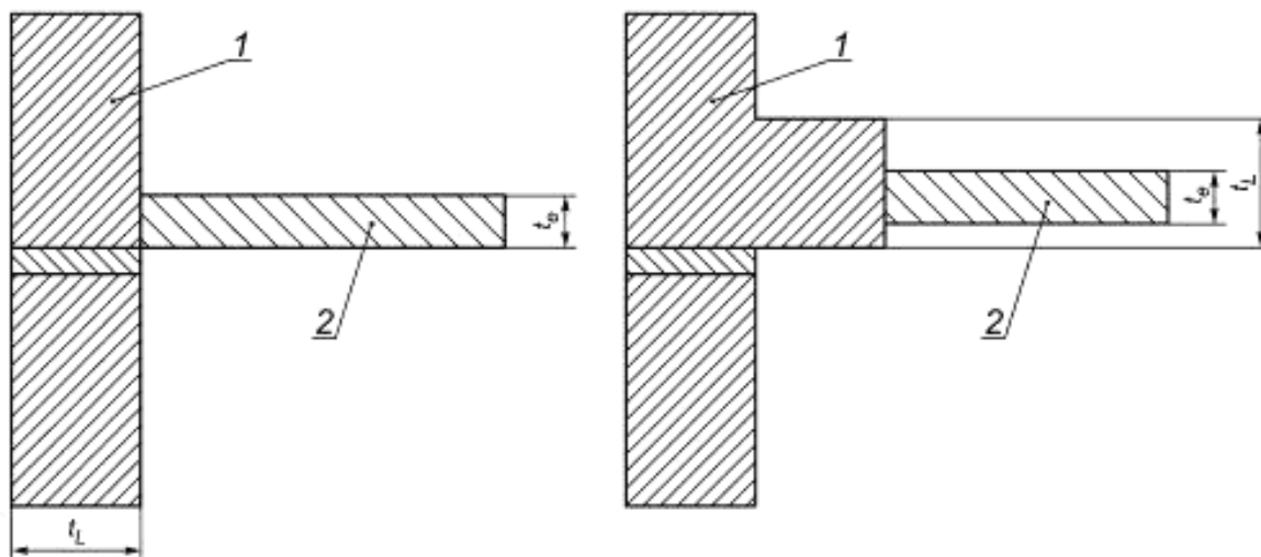
1 — стена испытательной установки; 2 — испытуемый объект; t_L — толщина стены испытательной установки; t_o — толщина испытуемого объекта
