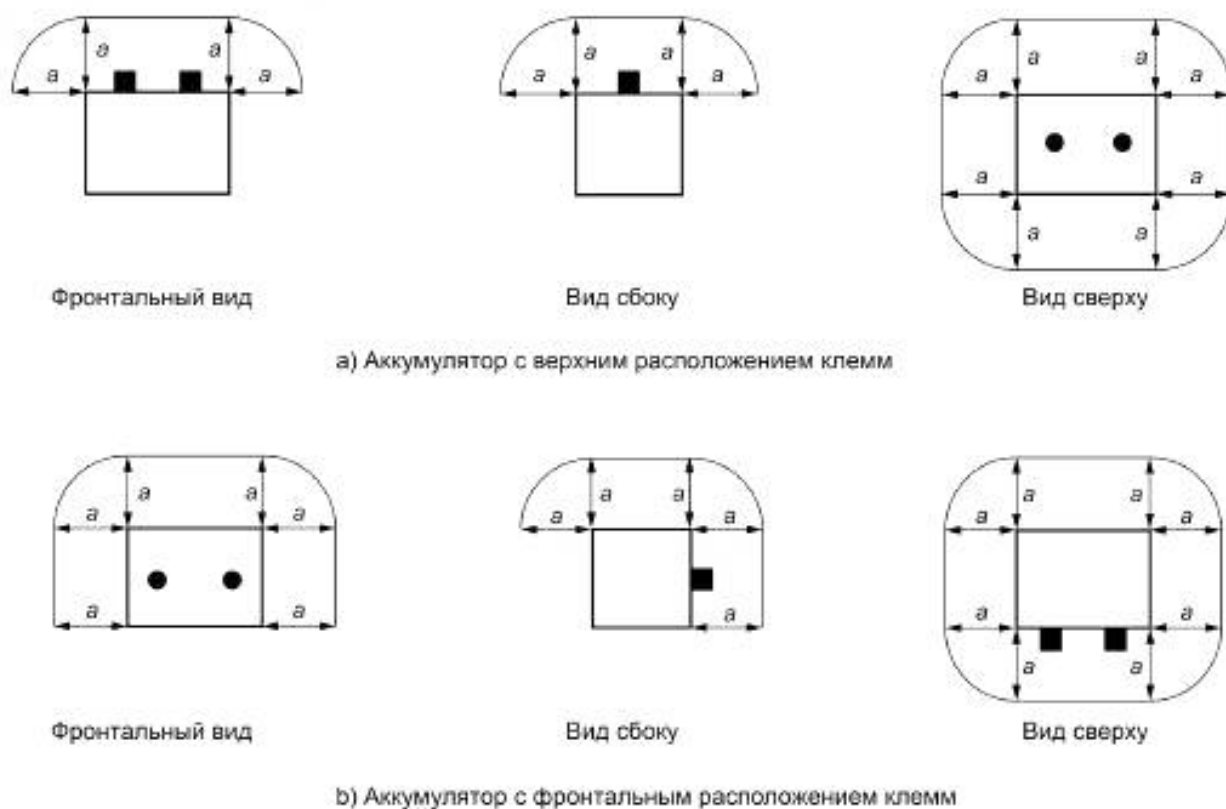
Рисунок 1 — Свободное пространство a вокруг аккумулятора
